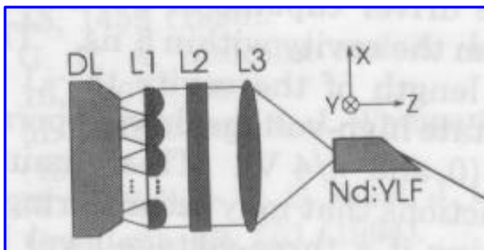
(a) 二极管直接端面泵浦固体激光器示意图
